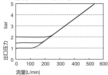
低压型溢流特性
