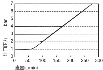
中压型溢流特性
