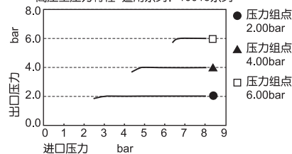
高压型压力特性 适用系列: 10015系列
