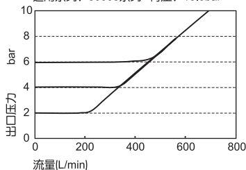
高压型溢流特性
