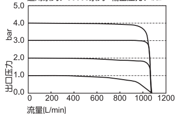
中压型流量特性
