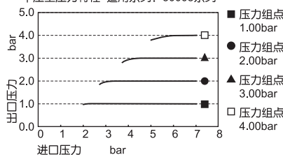
高压型压力特性 适用系列: 30008系列
