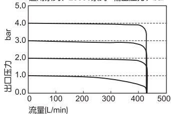
中压型流量特性
