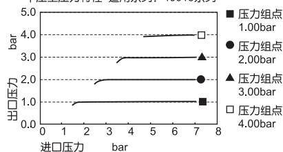
高压型压力特性 适用系列: 10015系列
