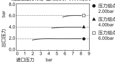
高压型压力特性 适用系列: 30008系列
