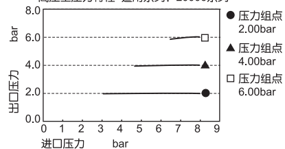
高压型压力特性 适用系列: 20006系列
